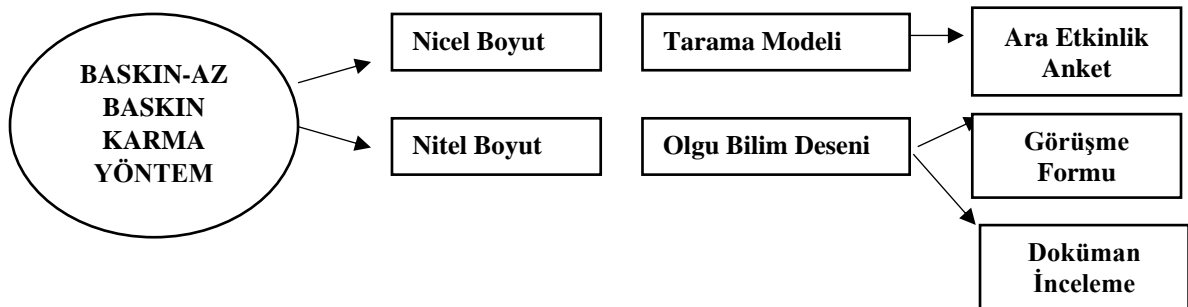
Şekil 1. Araştırma modeli
